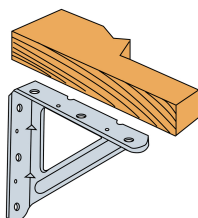
Fixation de console
