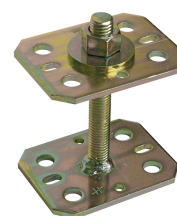
Petits pieds de poteau réglable APB7090
